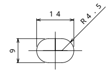
長丸穴詳細
